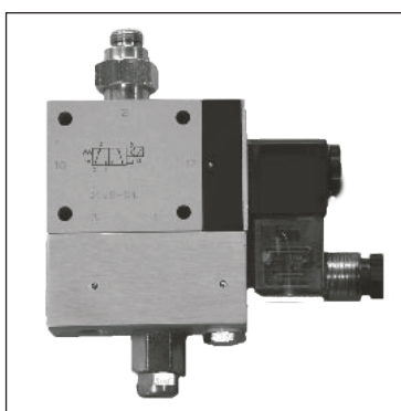
Układ zabezpieczający
